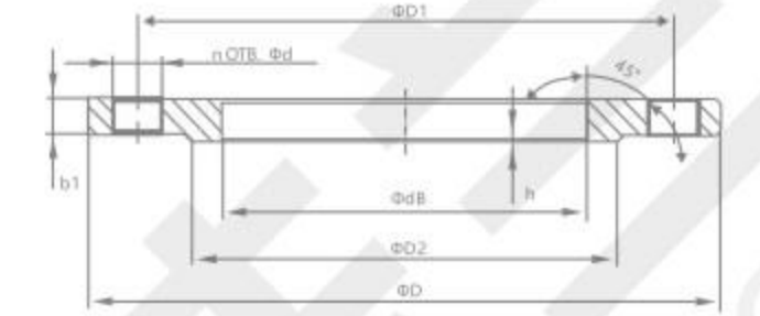
GOST 12821-80 平焊法兰
