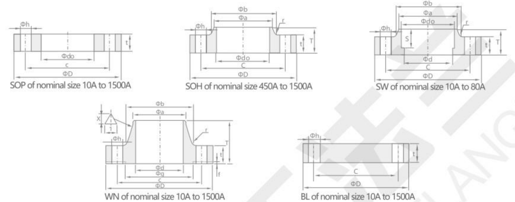
JIS B2220-2012(5K)
