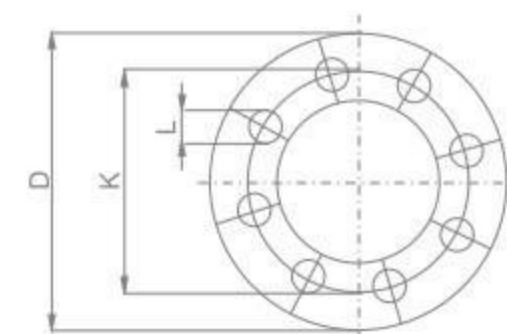
Dimensions of PN 16 Flanges EN 1092-1
