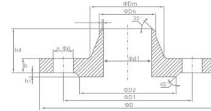
GOST 12820-80 带颈平焊法兰
